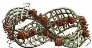
ruban de Möbius (MC Escher)
